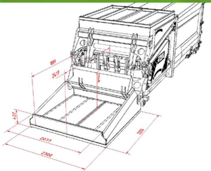
DECKELFUNKTION. In Transportstellung ist die Einfüllöffnung vollständig geschlossen.
